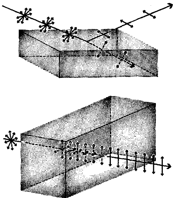
Поляризация света при отражении и прохождении через поляризующий кристалл
