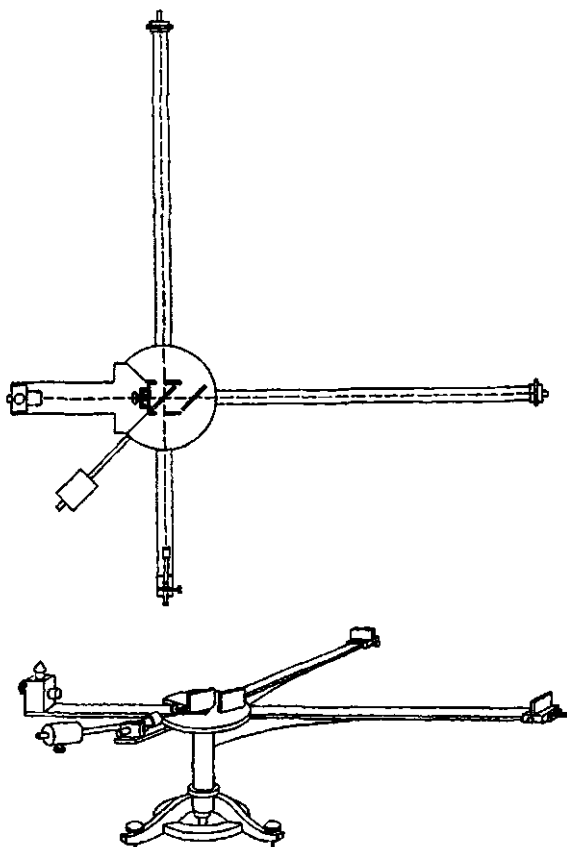
Первый интерферометр Майкельсона — вид сверху и сбоку
