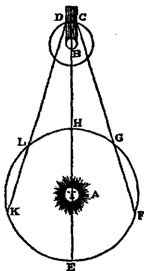
Схема Рёмера, изображающая затмение Юпитером (В) его спутника Ио (DC), наблюдаемое из различных точек земной орбиты (Земля вращается вокруг Солнца)
