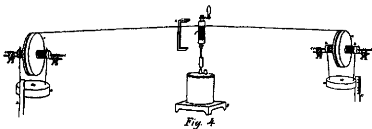
Усовершенствованная схема эксперимента Джоуля Рисунок из "Научных записок" Джоуля
