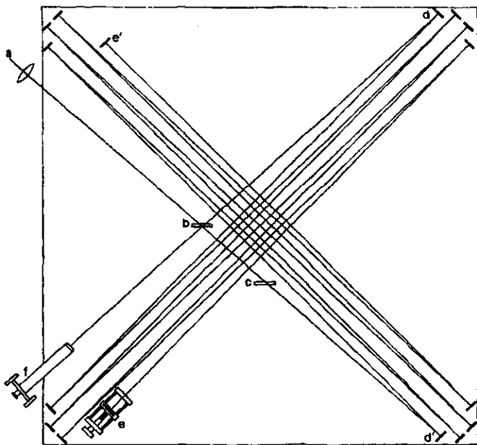
ЭКСПЕРИМЕНТ МАЙКЕЛЬСОНА-МОРЛИ. НА НИЖНЕЙ СХЕМЕ ПОКАЗАНО, КАК ПРОХОДИЛИ ДВА СВЕТОВЫХ ПУЧКА, ПУТЬ КОТОРЫХ БЫЛ УВЕЛИЧЕН ОТРАЖЕНИЕМ ОТ ШЕСТНАДЦАТИ ЗЕРКАЛ
