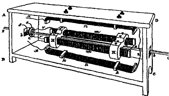
Электрический мотор Джоуля Рисунок из его "Научных записок"
