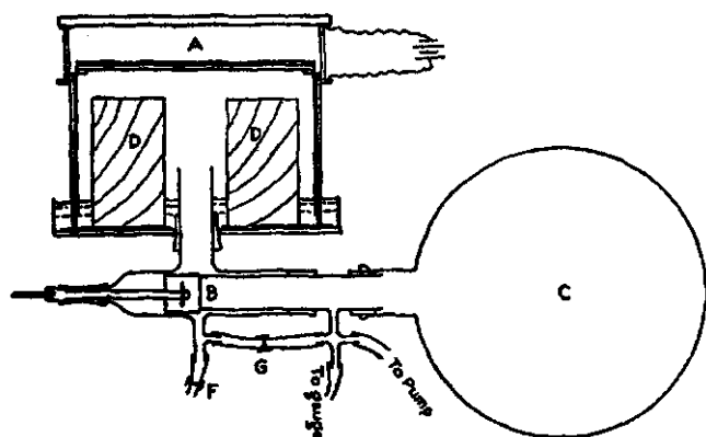
Ионизационная камера Вильсона. Вакуум С при открытии впускного клапана В всасывает через основание камеры А находящийся в ней влажный воздух. Увеличение объема ведет к образованию облака
