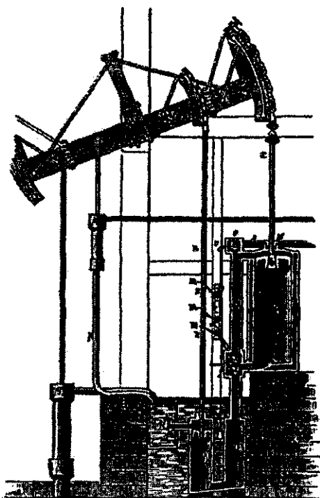
ПАРОВАЯ МАШИНА, СОЗДАННАЯ В КОНЦЕ XVIII ВЕКА ДЖЕЙМСОМ УАТТОМ
