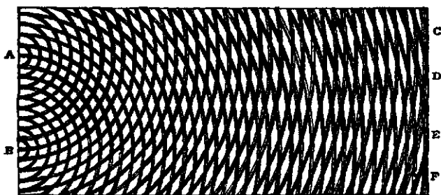
КАРТИНКА ИНТЕРФЕРЕНЦИИ, ПОЛУЧЕННАЯ ТОМАСОМ ЮНГОМ
