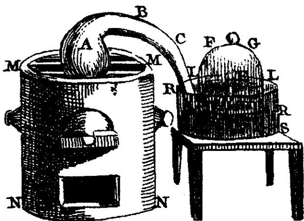
НАГРЕВ РТУТИ В КОЛБЕ, ВЫПОЛНЕННОЙ В ФОРМЕ "ФЛАМИНГО" Рисунок Марии-Анны Лавуазье
