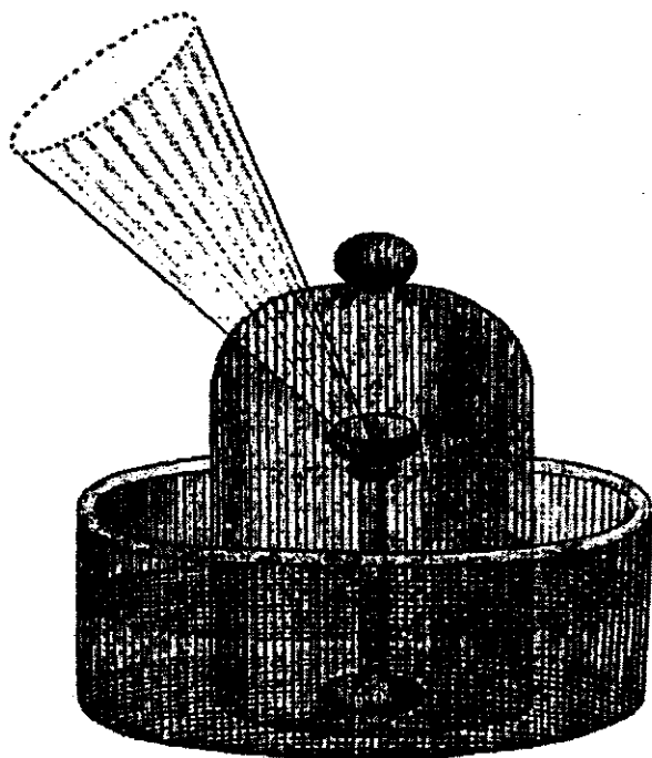
СЖИГАНИЕ ОКСИДА СВИНЦА В СТЕКЛЯННОМ СОСУДЕ С ПОМОЩЬЮ УВЕЛИЧИТЕЛЬНОГО СТЕКЛА
