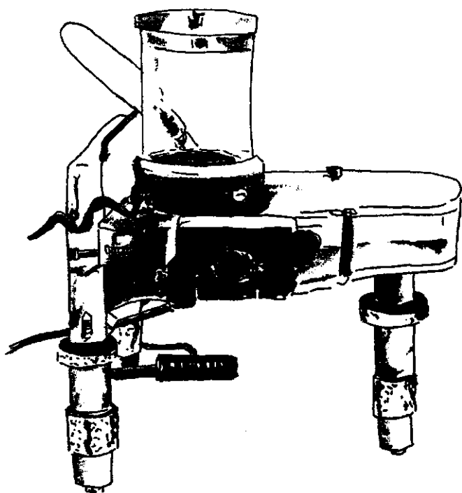
Установка Милликена производства компании Phillip Harris Рисунок Элисон Кент
